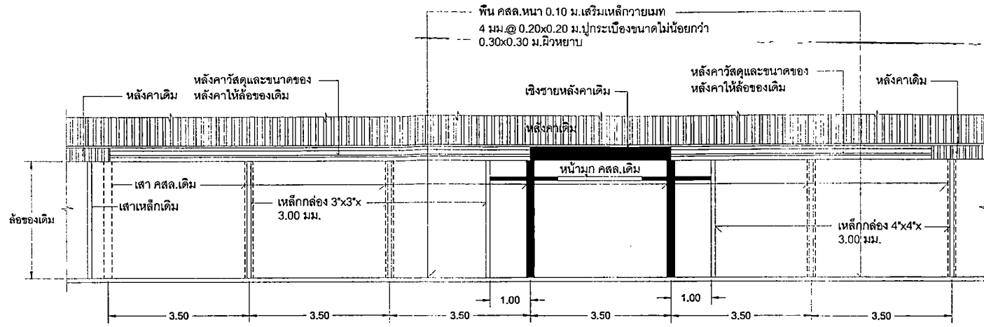
รูปตัด 1 - 1
