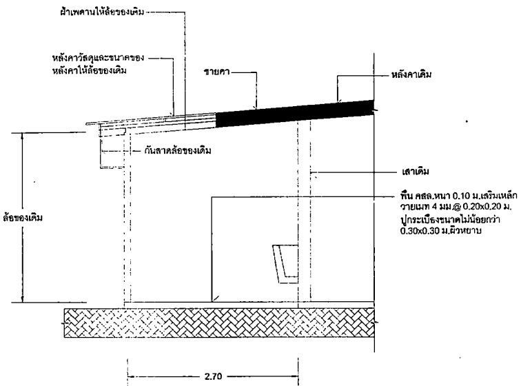
รูปตัด 3 - 3
