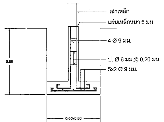
ขยาย F1
